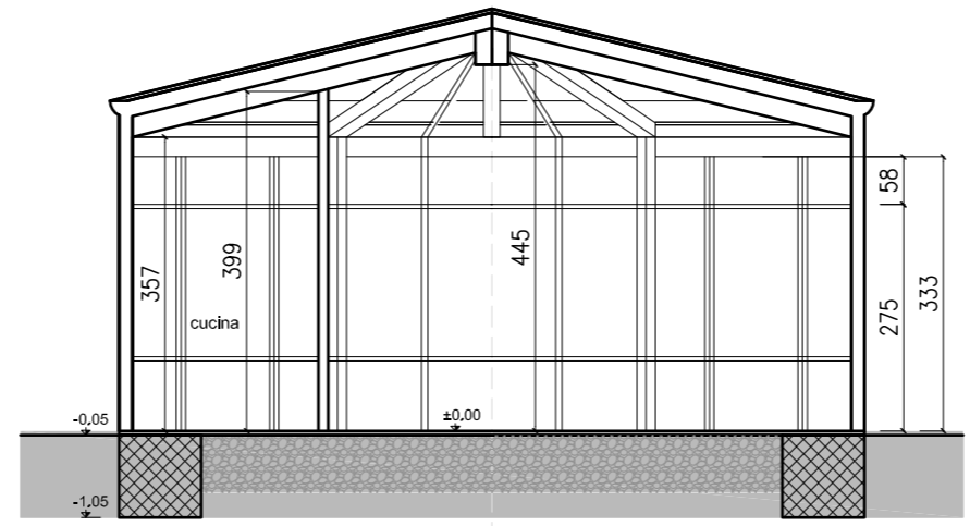
sezione AA
