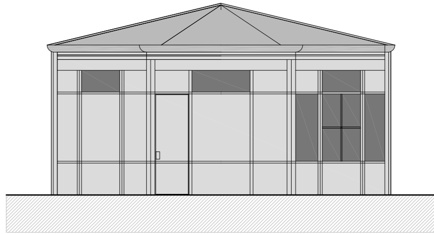
prospetto est
