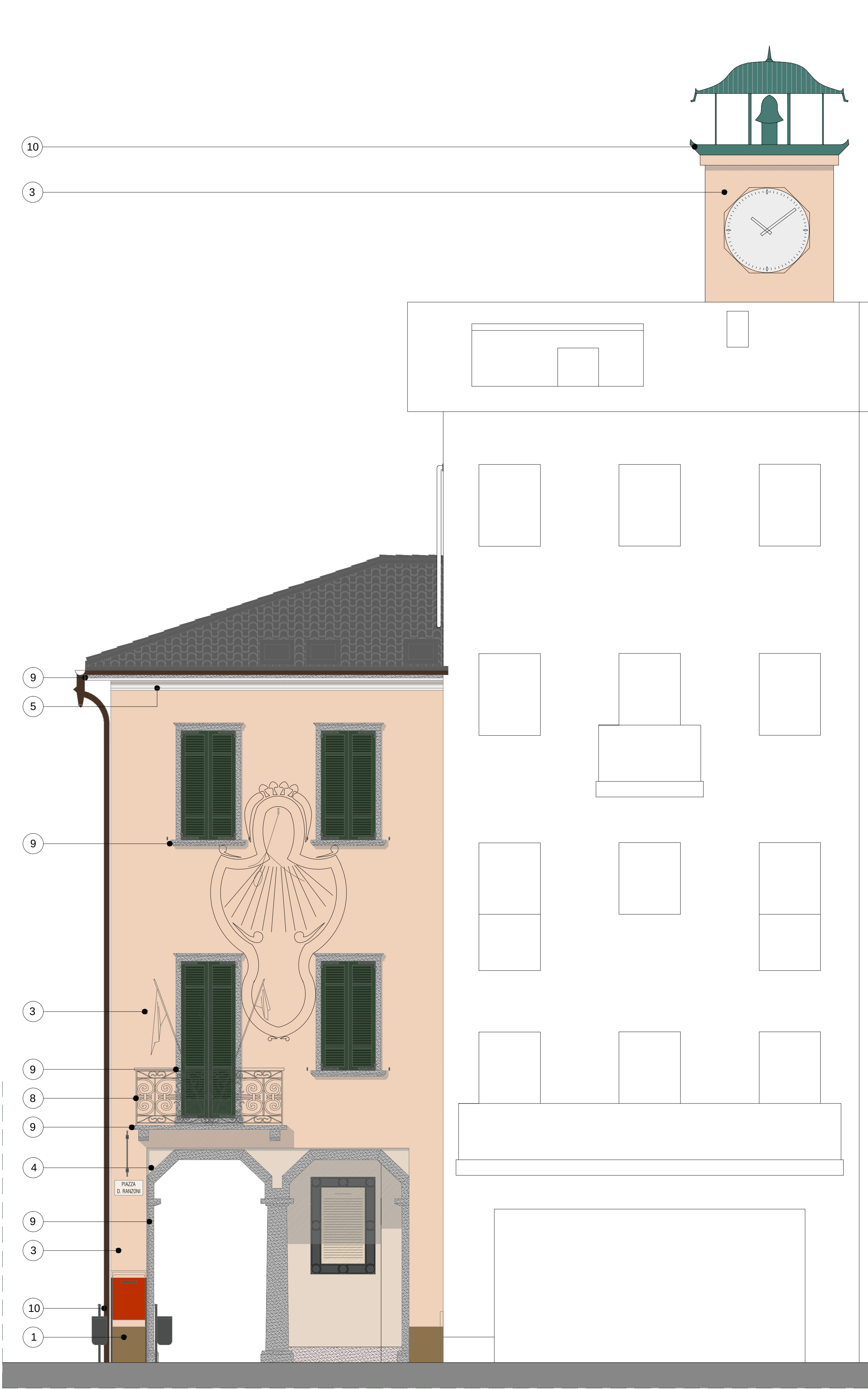
PROSPETTO SUD
