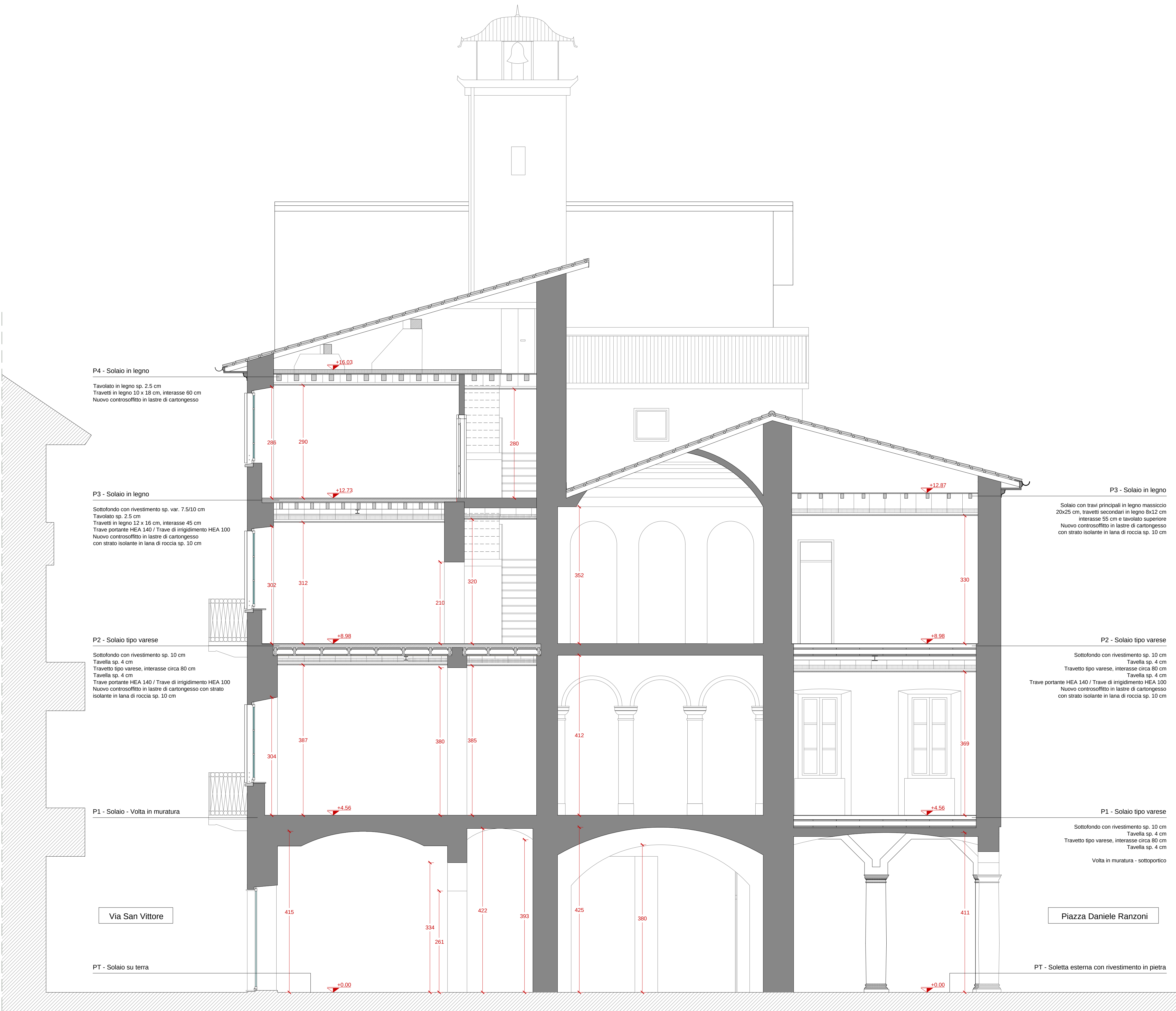
SEZIONE AA
