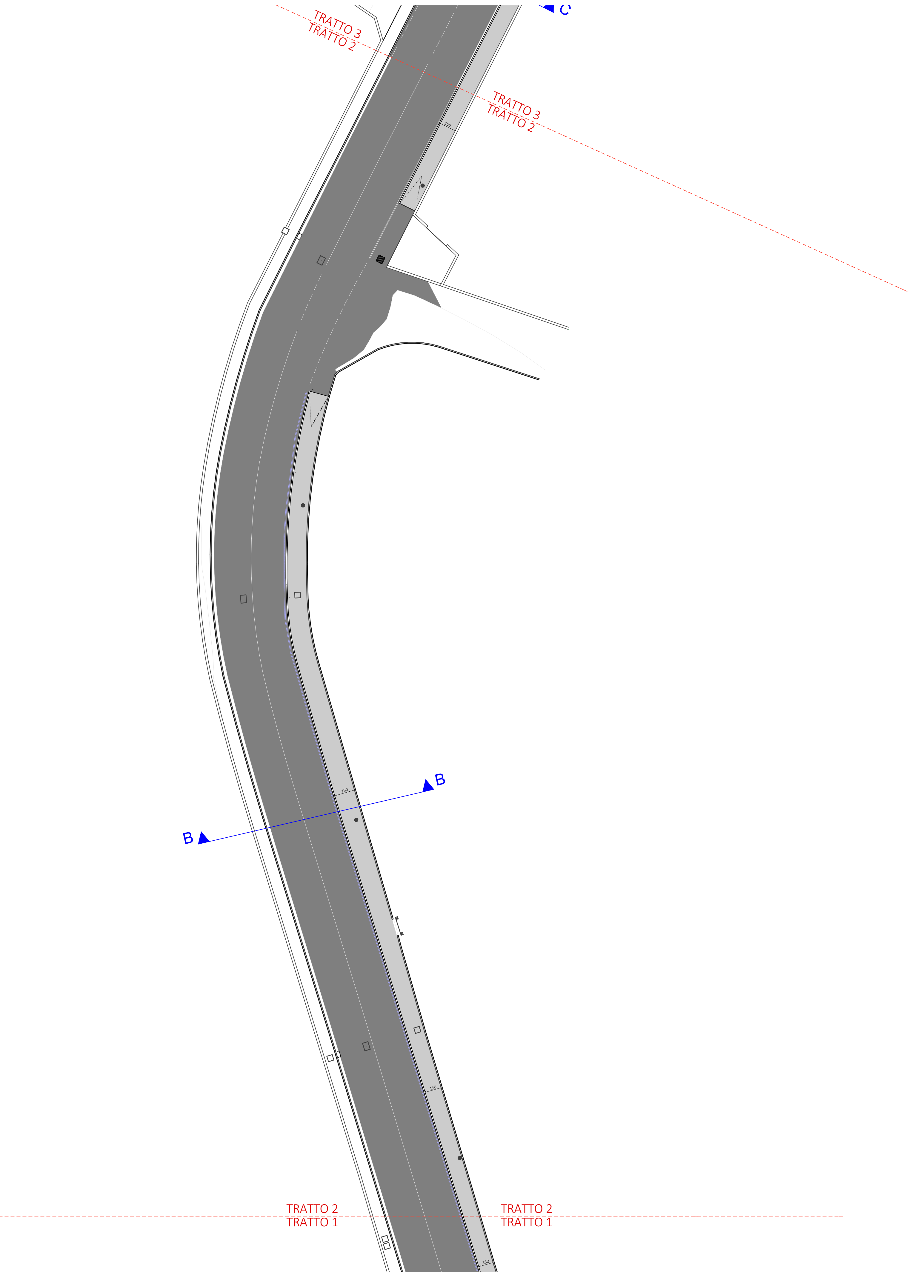
PLANIMETRIA DI PROGETTO TRATTO 2 >> Scala 1:200
