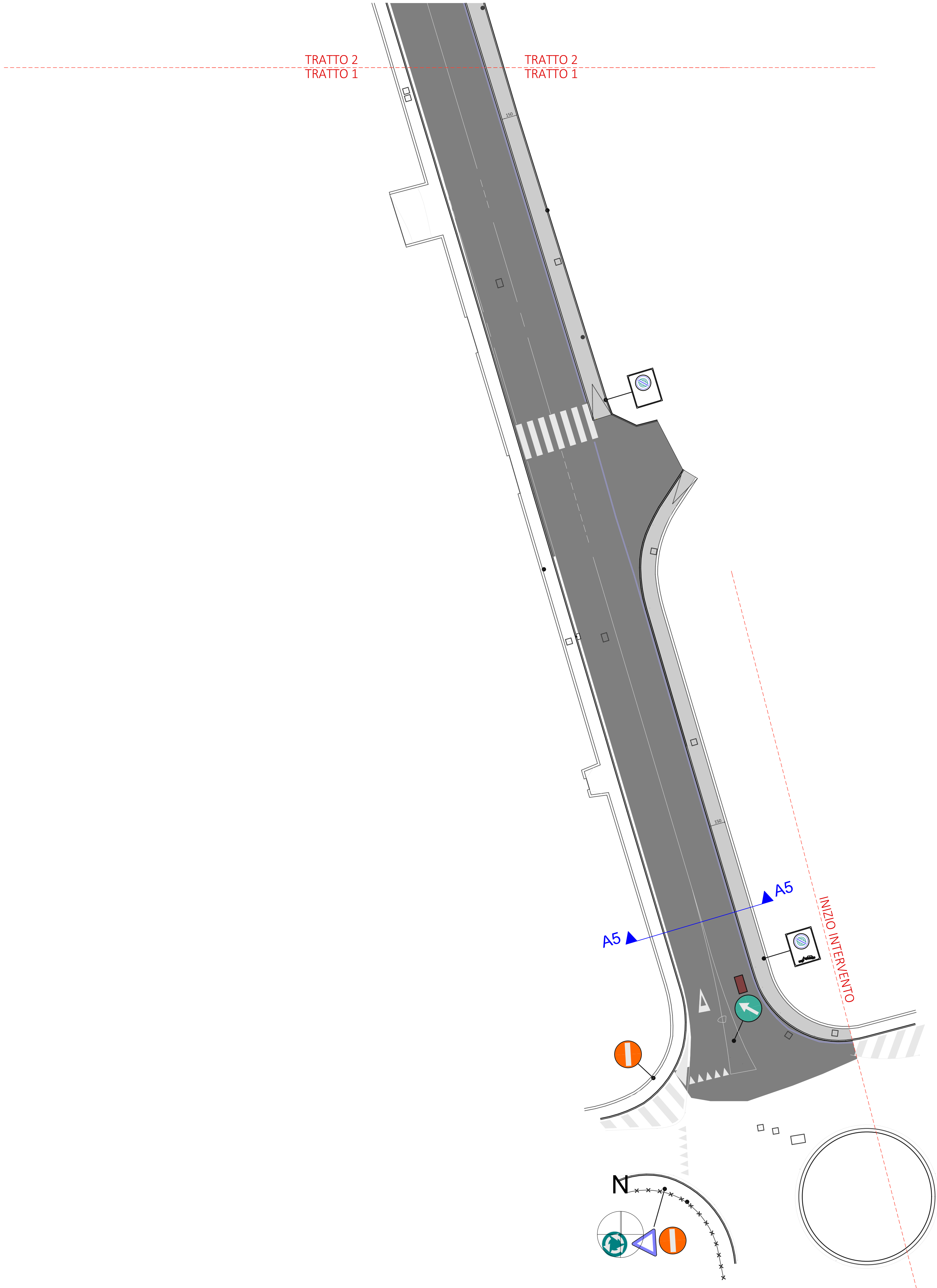
PLANIMETRIA DI PROGETTO TRATTO 1 >> Scala 1:200
